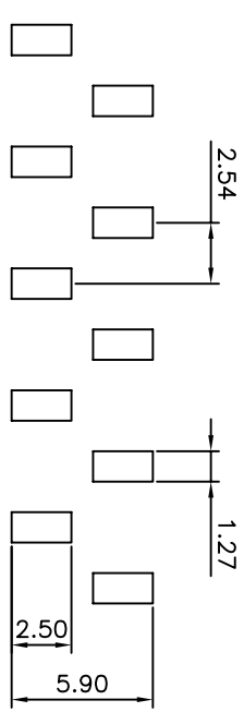
P.C.B LAYOUT
