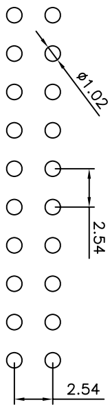
P.C.B LAYOUT
