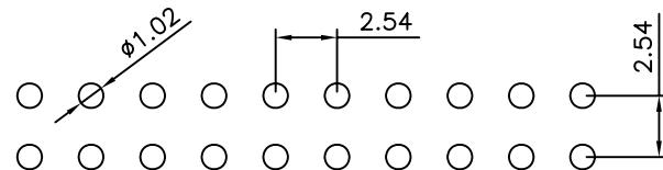
P.C.B LAYOUT
