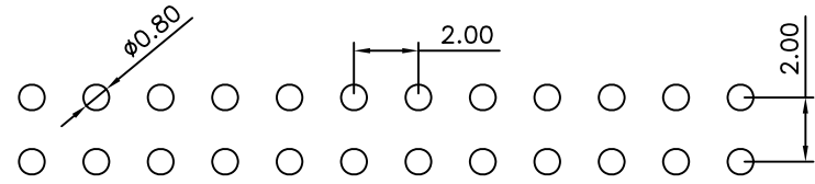
P.C.B LAYOUT
