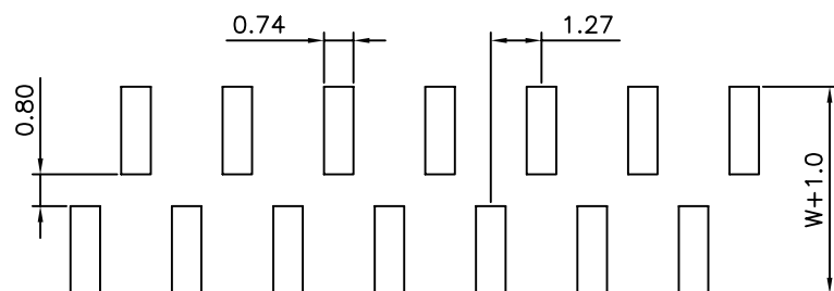
P.C.B LAYOUT
