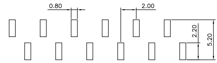
P.C.B LAYOUT
