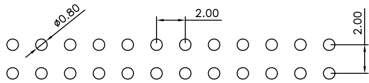
P.C.B. LAYOUT
