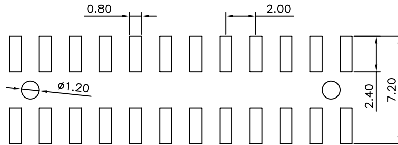
P.C.B LAYOUT
