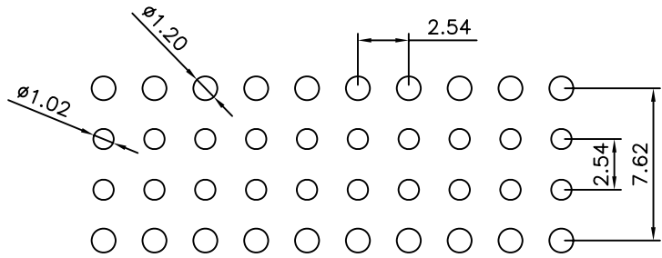
P.C.B LAYOUT
