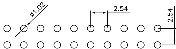
P.C.B LAYOUT
