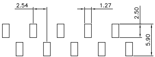
P.C.B LAYOUT
